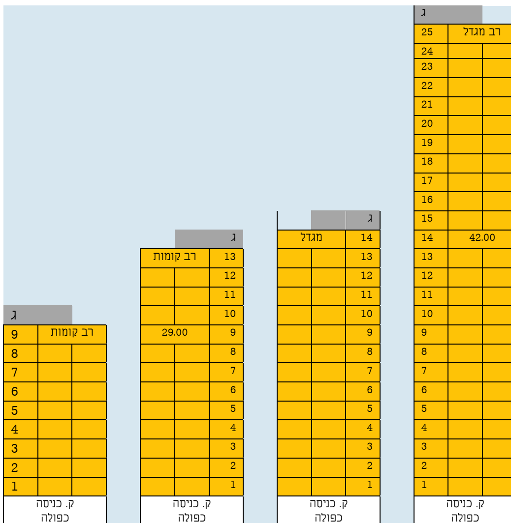
נפחי בניה אפשריים בקטגוריית רבי קומות ומגדלים מקרא - צהוב: קומה תב"עית / אפור בהיר: בניה על הגג
